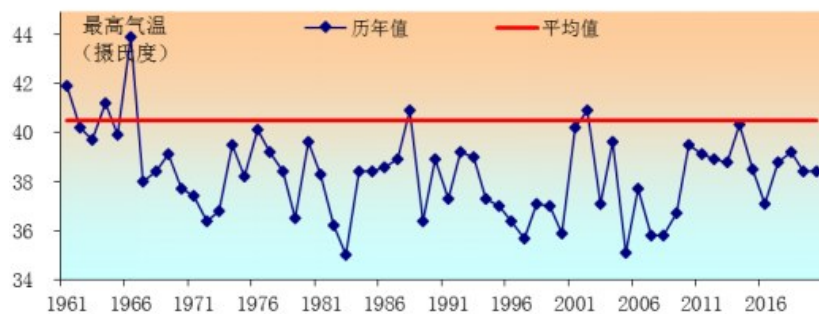
图2:1961—2020年7月平均最高气温历年变化曲线(℃)
