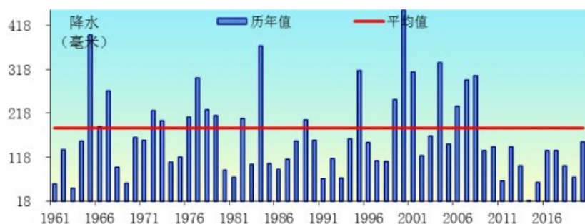
图3:1961—2020年7月降水历年变化曲线(毫米)
