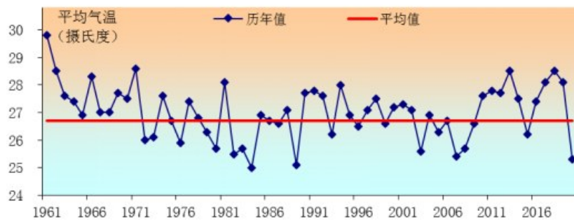
图1:1961—2020年7月平均气温历年变化曲线(℃)
