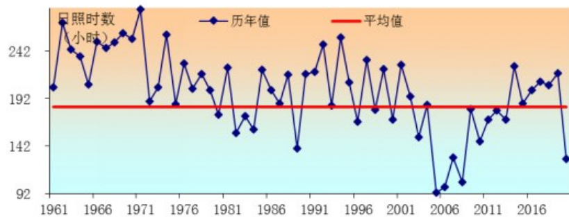
图4:1961—2020年7月平均日照时数历年变化曲线(小时)
