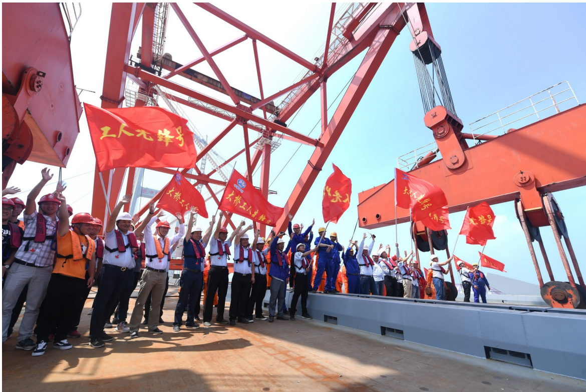
6月5日,福平铁路平潭海峡公铁两用大桥元洪航道桥主桥成功合龙,为下一步福平铁路全线贯通提供有力保障。元洪航道桥为双塔双索面钢桁混合梁斜拉桥,全桥长1188米,其中主跨达532米。
