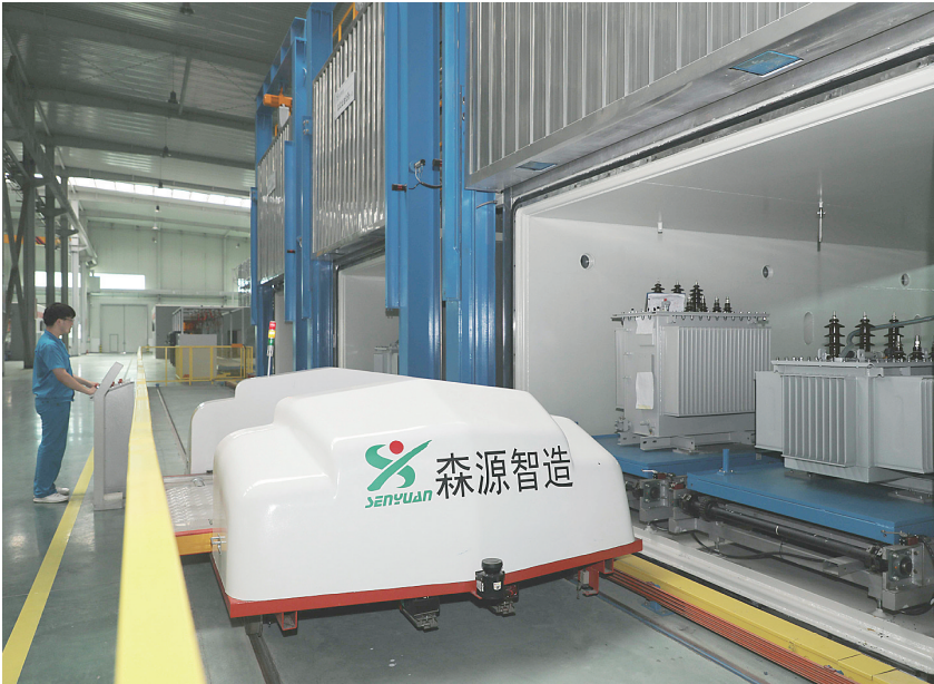
图为森源电气智能型节能变压器柔性制造系统全过程使用RGVAGV机器人自动输送,最终实现产品自动入库。
